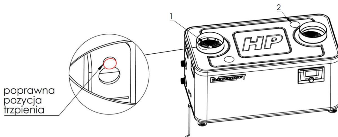
Rys. 5b. Instalacja pompy ciepła na wieszakach.
