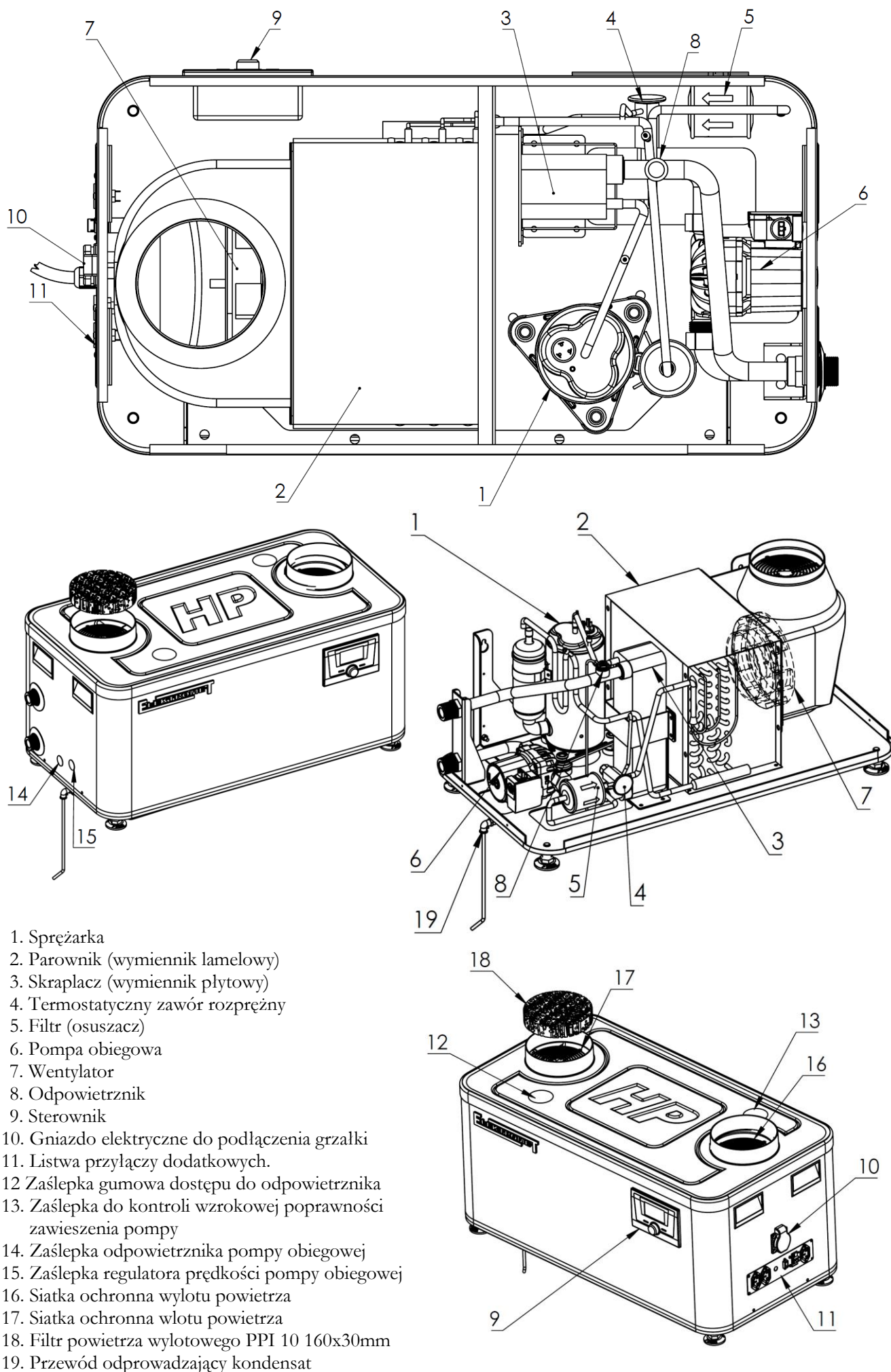
Rys. 2. Budowa pompy ciepła HP ALFA 2.4
