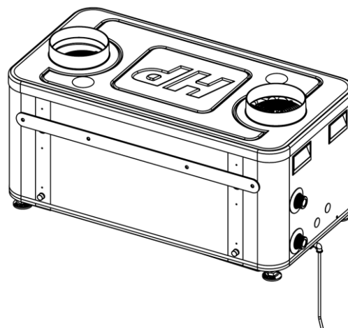
Rys. 5a. Instalacja pompy ciepła na wieszakach.
