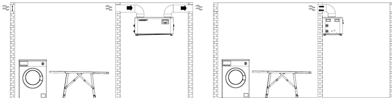
Rys. 8. Przykłady instalacji pompy ciepła.
