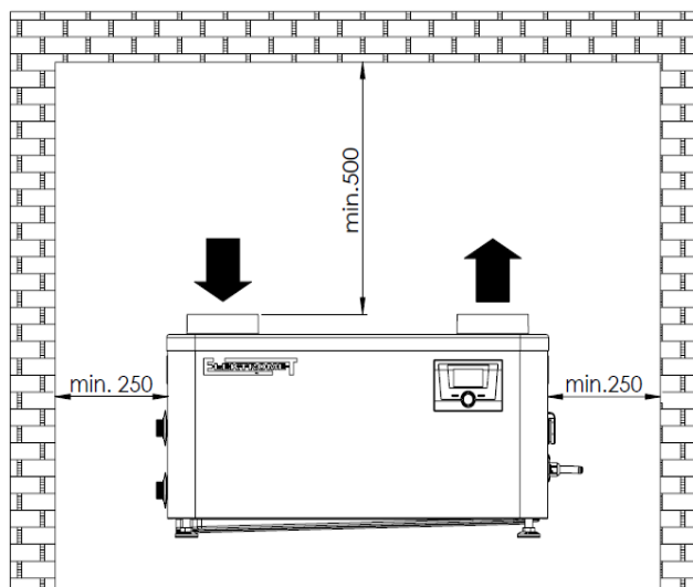
Rys. 4. Instalacja pompy ciepła z zachowaniem niezbędnych odstępów.
